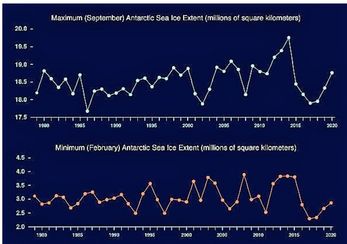
Évolution des minima et maxima des glaciers Pôle Sud sur une longue période
